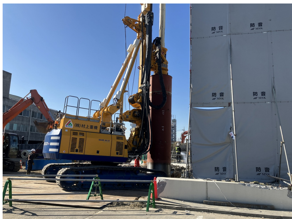
地下躯体撤去（トレンチ）
