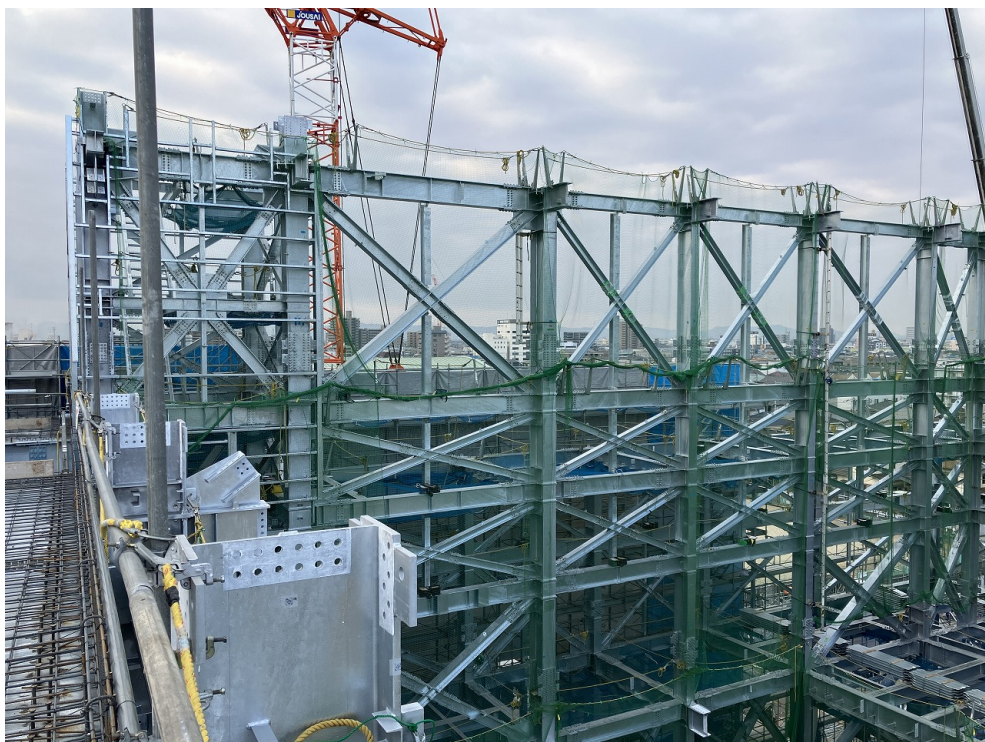
3工区鉄骨建方
