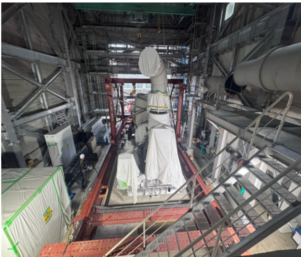
蒸気タービンおよび発電機
