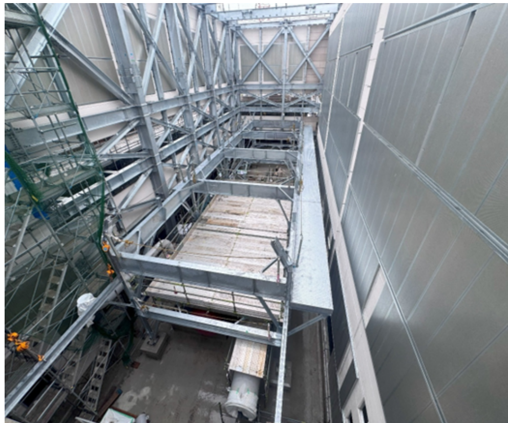
復水器エリア架台および歩廊組立
